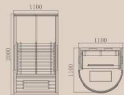
04-K1 Size: 1100×1100×2000mm
