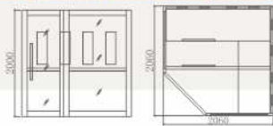
05-K10 Size: 2060×2060×2000mm
